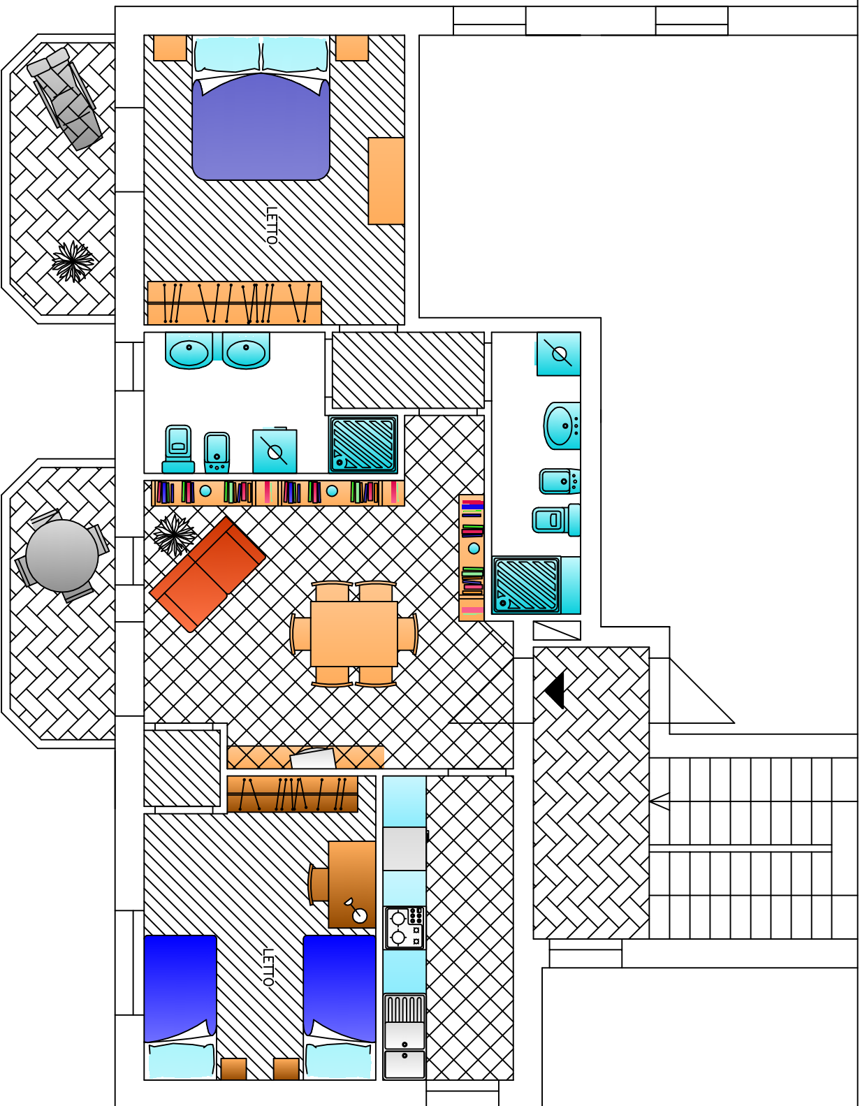
PIANTA PIANO SECONDO ALLOGGIO N.5
